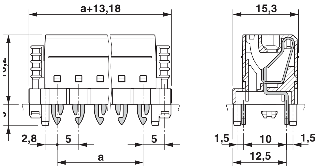
Rysunek wymiarowy
