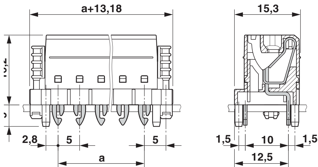
Rysunek wymiarowy
