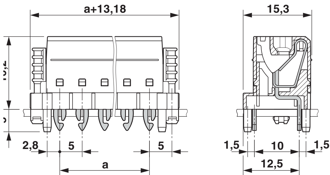
Rysunek wymiarowy
