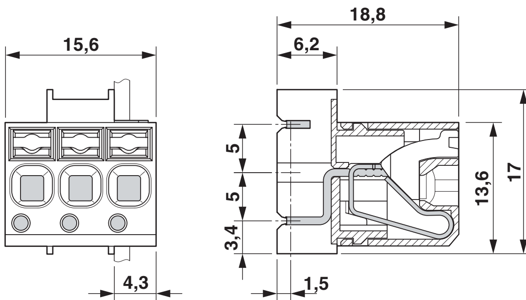
Rysunek wymiarowy
