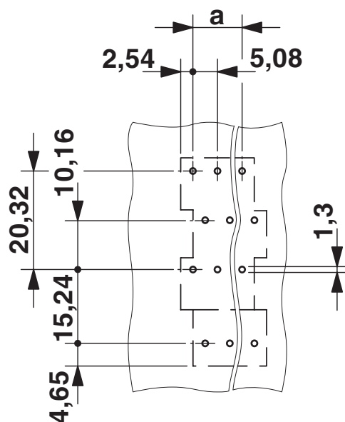
Rysunek wymiarowy
