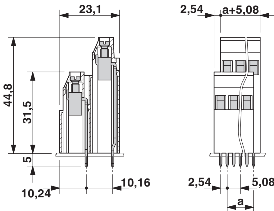
Rysunek wymiarowy wersji 3-biegunowej produktu
