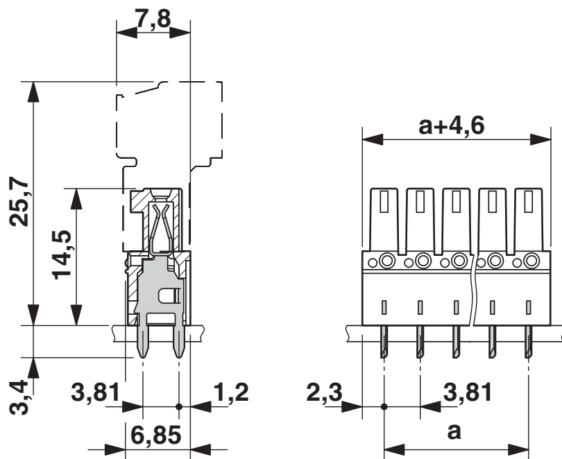
Rysunek wymiarowy
