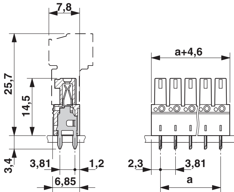
Rysunek wymiarowy
