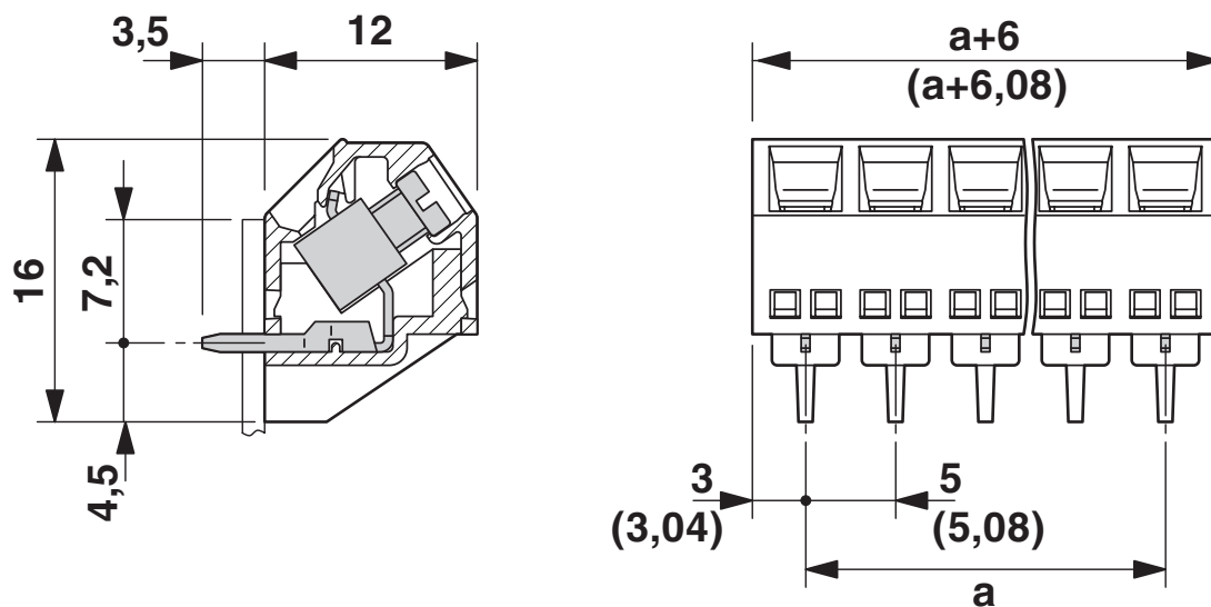
Rysunek wymiarowy
