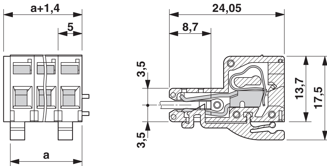
Rysunek wymiarowy
