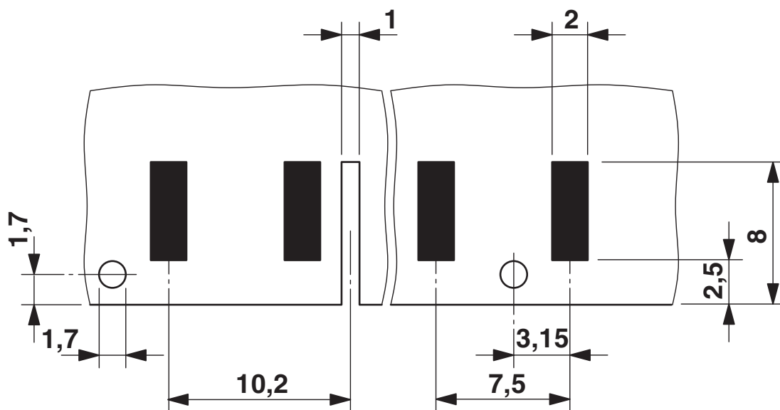
Otworowanie/geometria płytek lutowniczych
