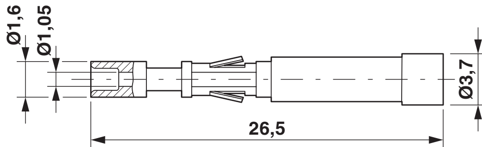
Rysunek wymiarowy
