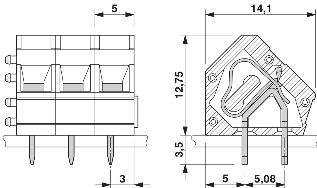
Rysunek wymiarowy
