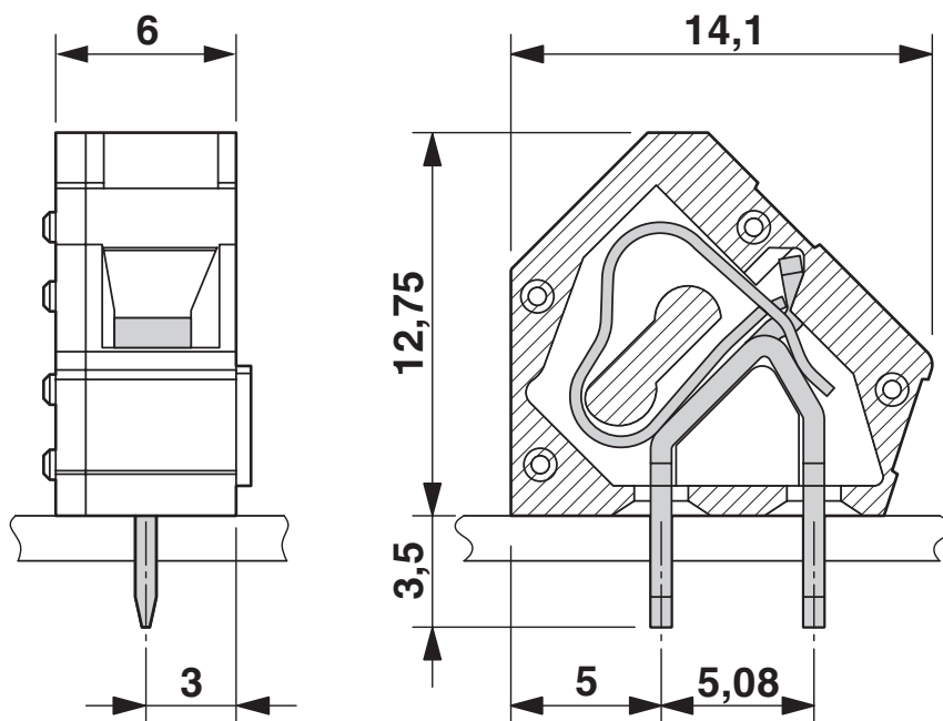
Rysunek wymiarowy
