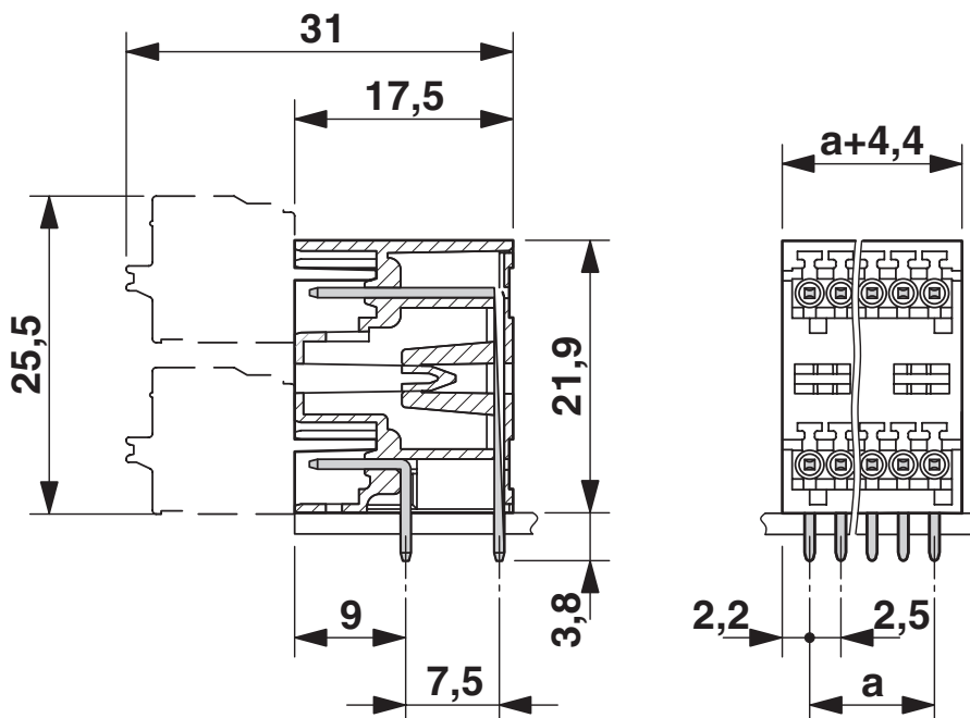
Rysunek wymiarowy
