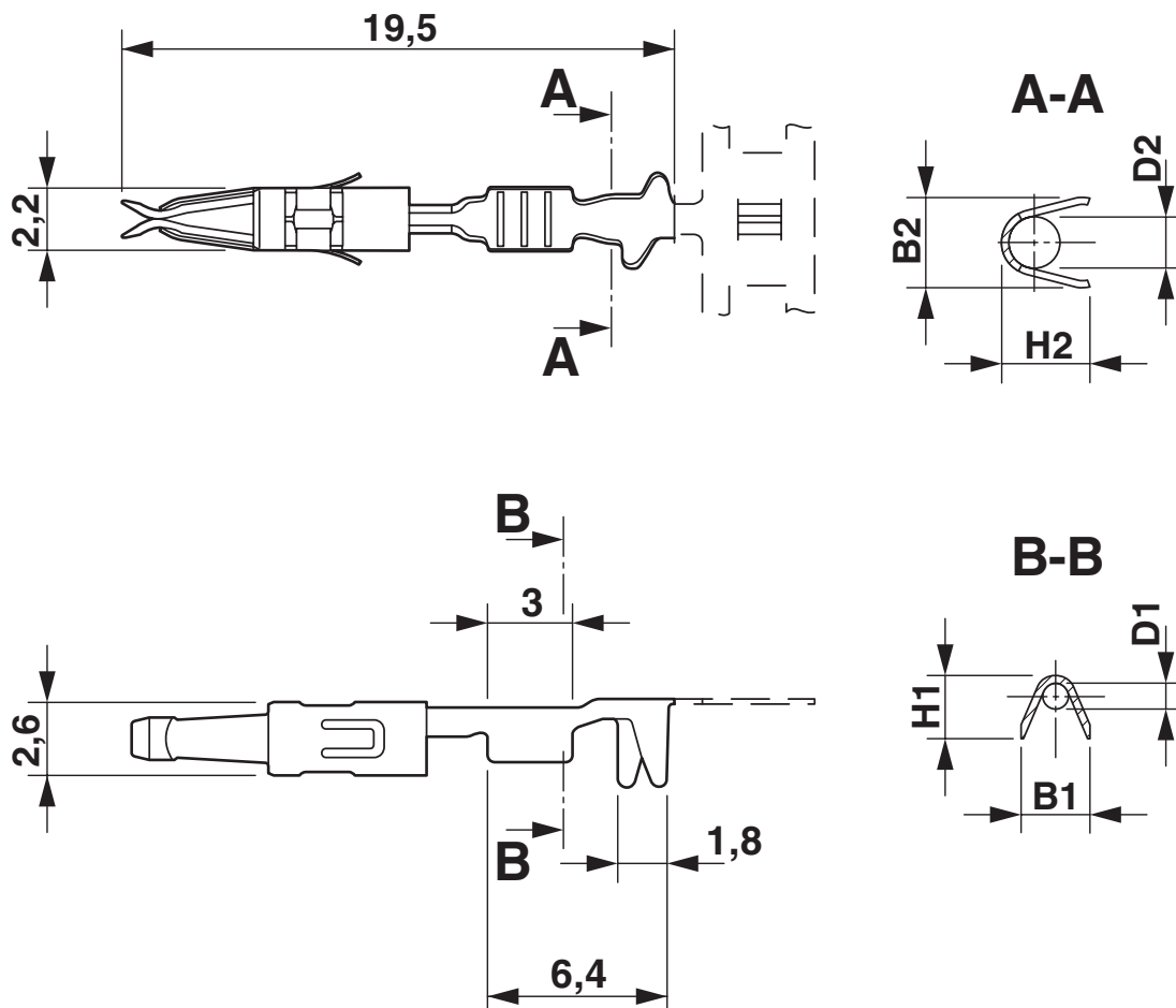
Rysunek wymiarowy
