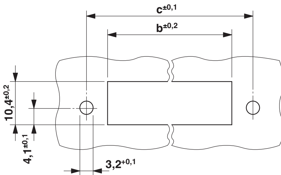
Rysunek wymiarowy
