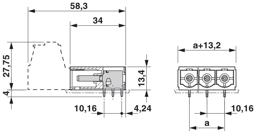
Rysunek wymiarowy
