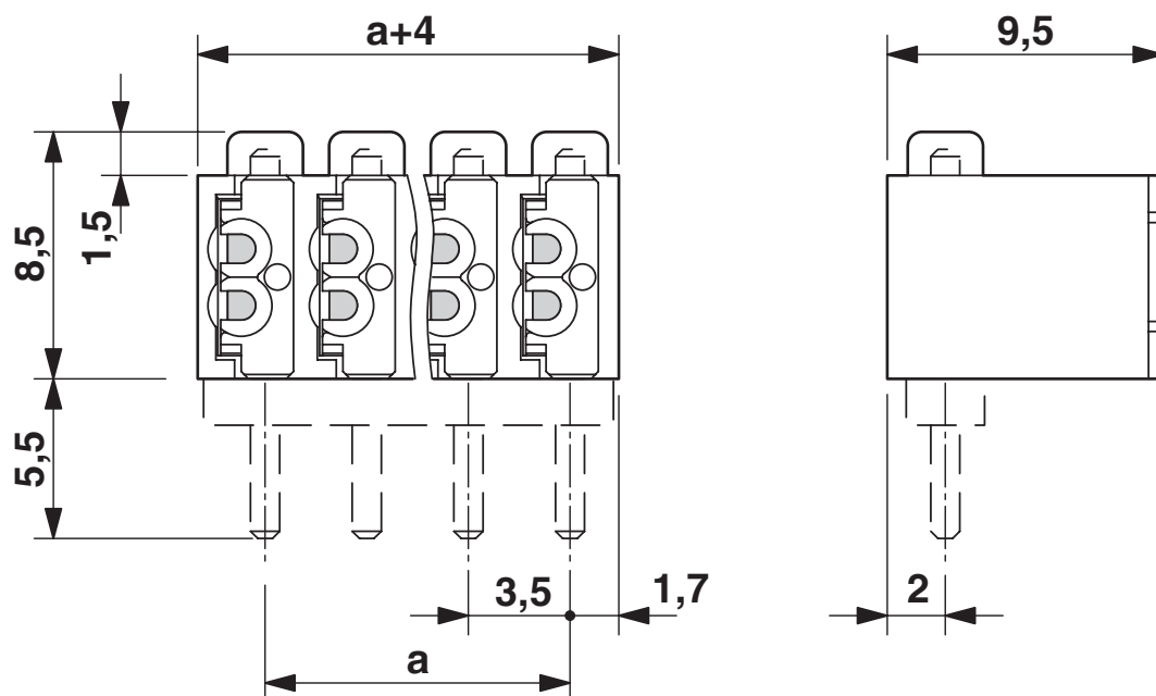
Rysunek wymiarowy
