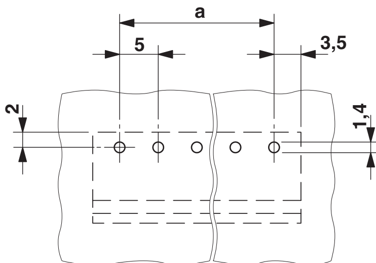
Otworowanie/geometria płytek lutowicznych
