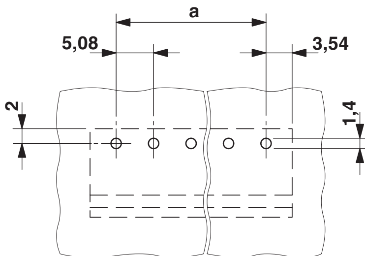
Rysunek wymiarowy
