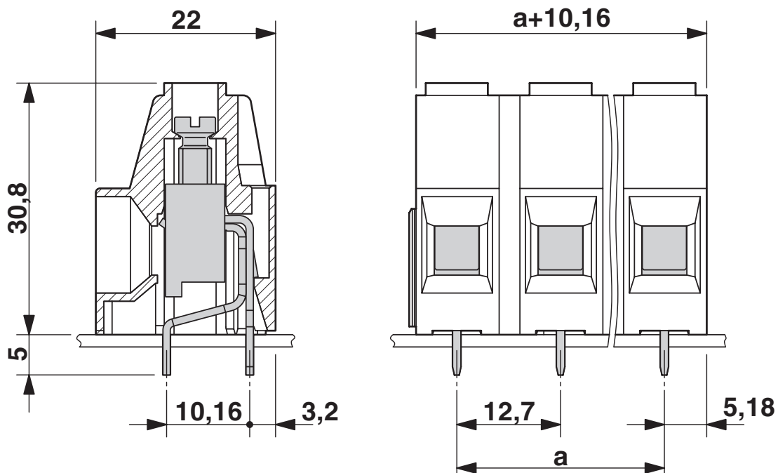
Rysunek wymiarowy
