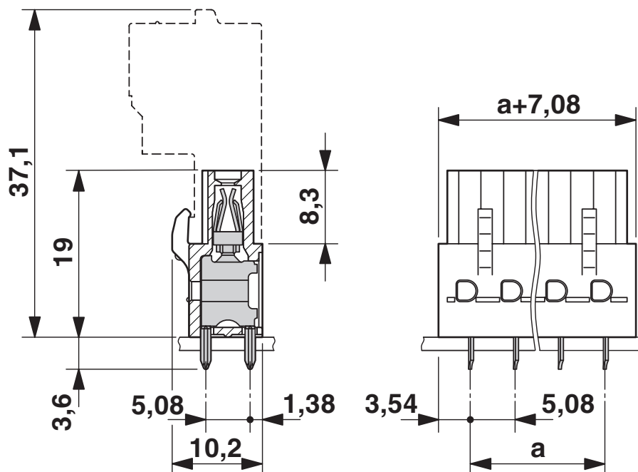
Rysunek wymiarowy
