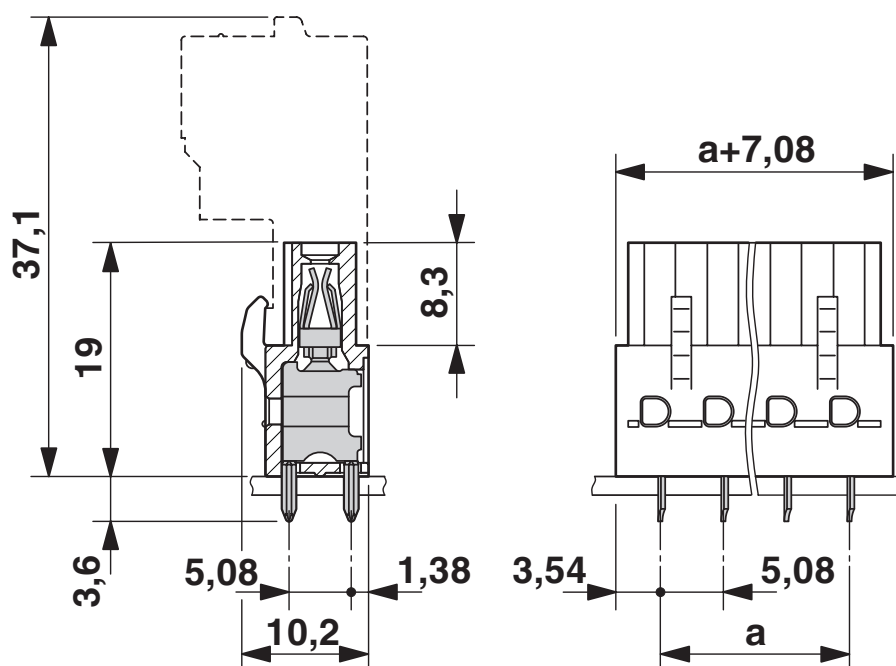
Rysunek wymiarowy
