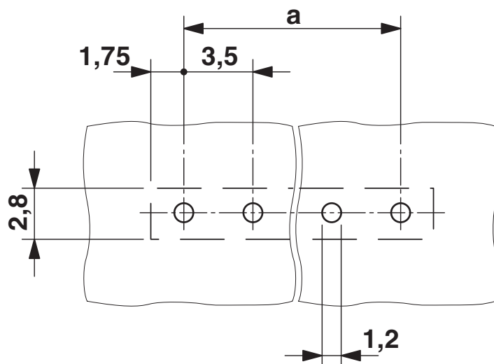
Rysunek wymiarowy
