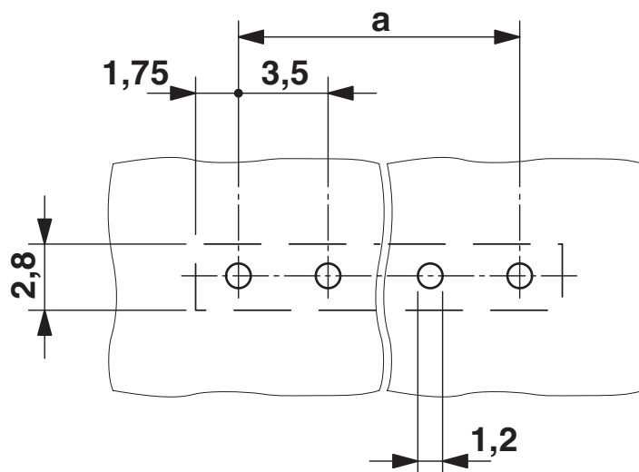
Rysunek wymiarowy
