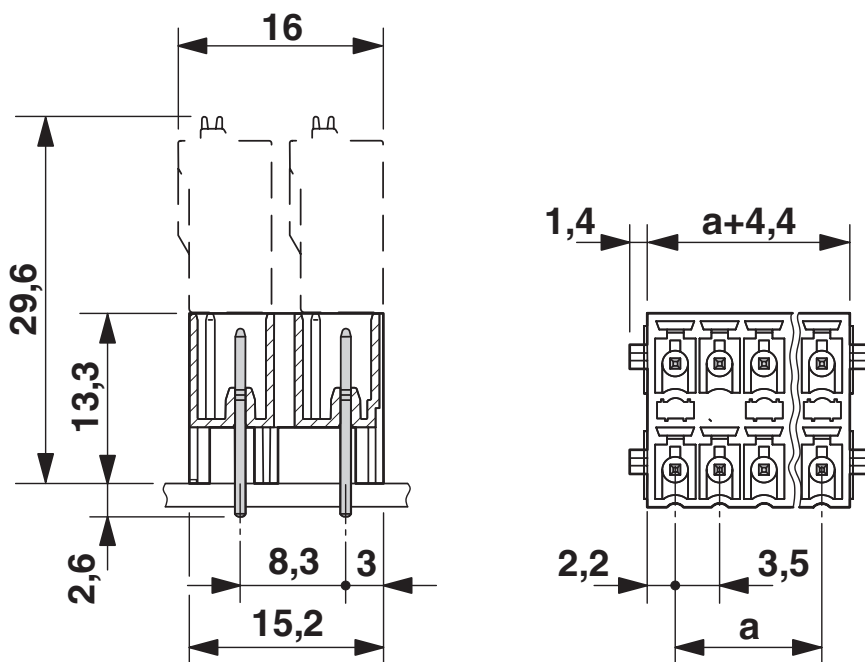
Rysunek wymiarowy
