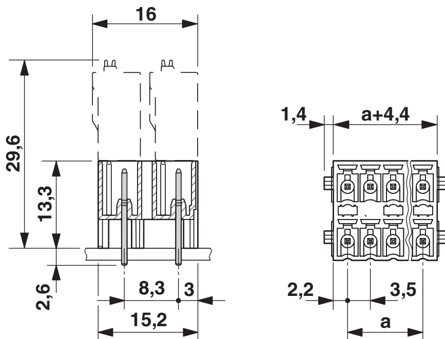
Rysunek wymiarowy
