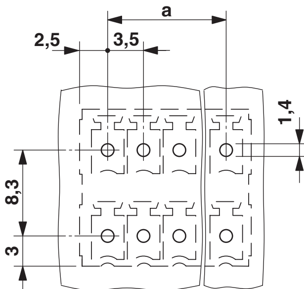
Otworowanie/geometria płytek lutowiczych
