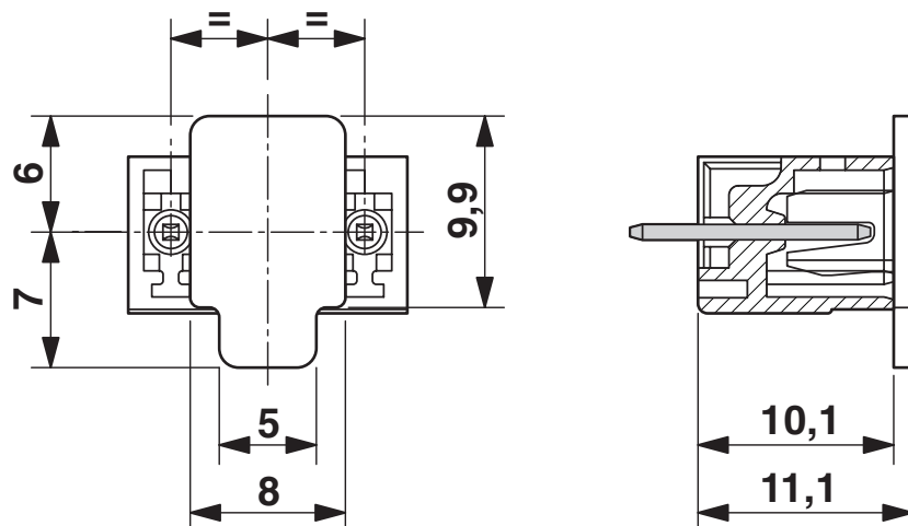
Rysunek wymiarowy
