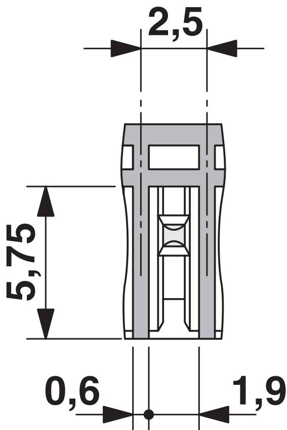
Rysunek wymiarowy
