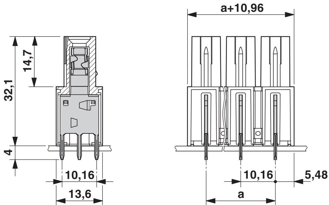
Rysunek wymiarowy
