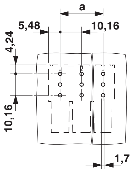
Rysunek wymiarowy
