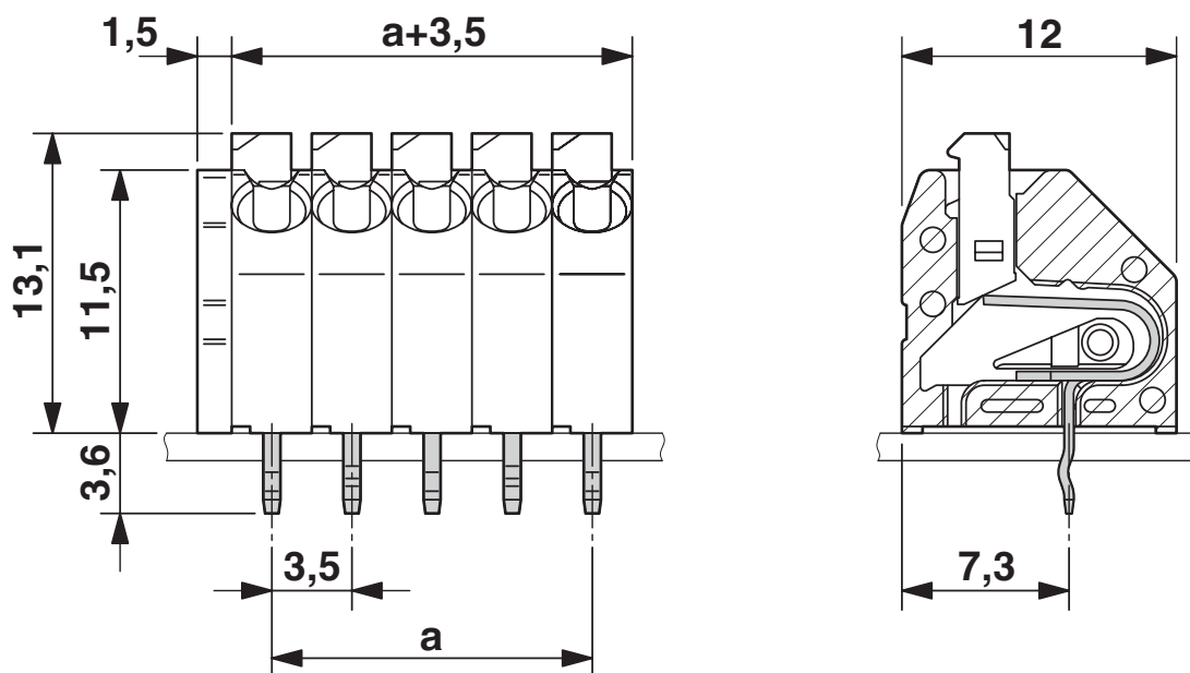
Rysunek wymiarowy
