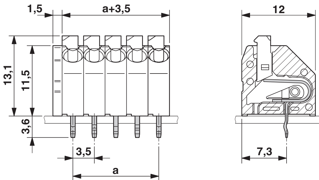
Rysunek wymiarowy wersji 5-biegunowej produktu
