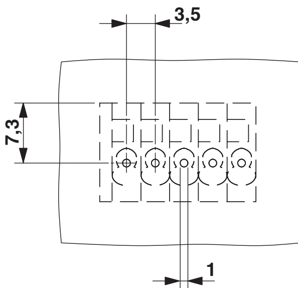
Rysunek pokazuje otworowanie dla wersji 5-biegunowej produktu
