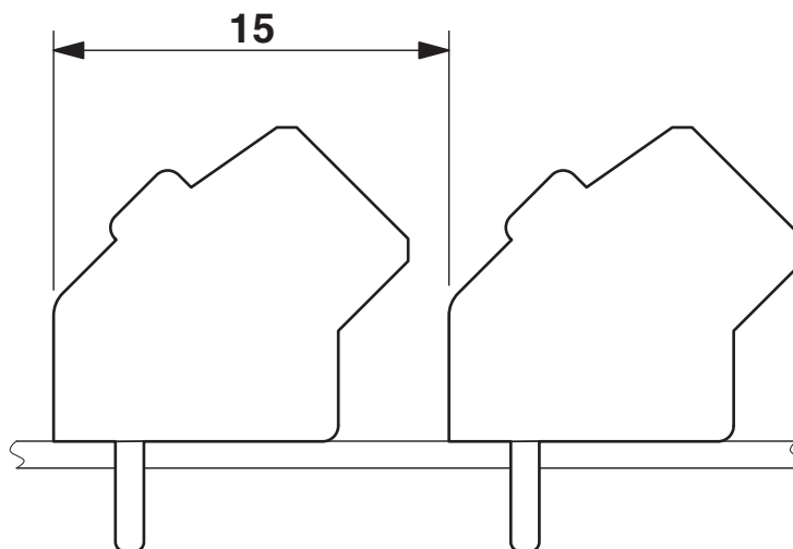
Rysunek wymiarowy
