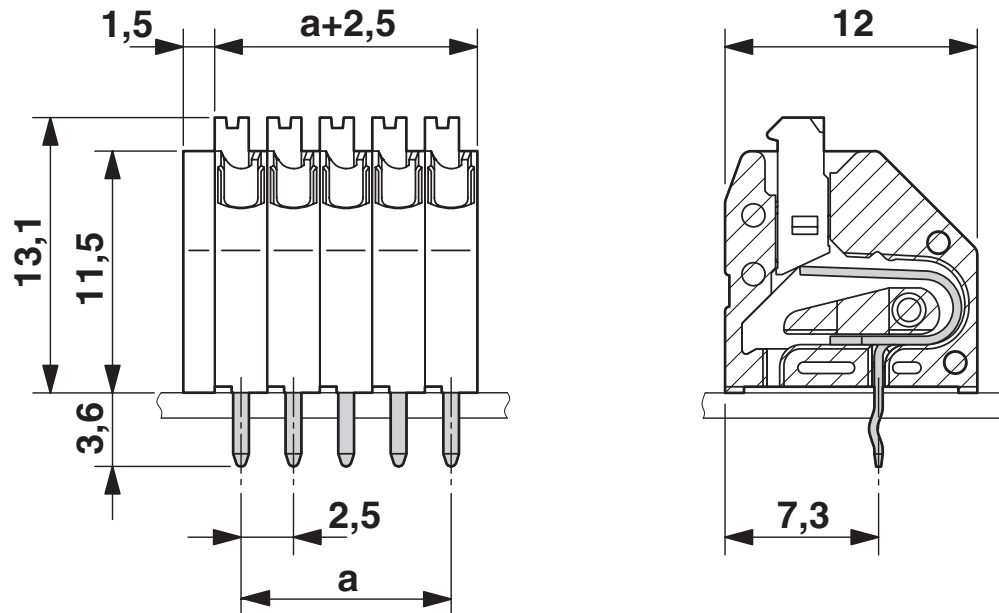
Rysunek wymiarowy
