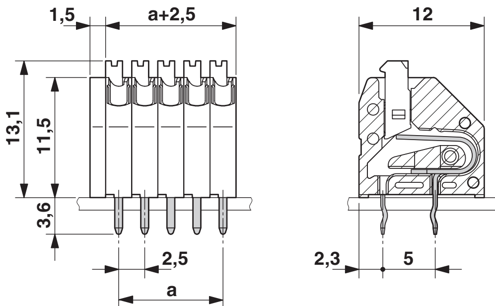
Rysunek wymiarowy
