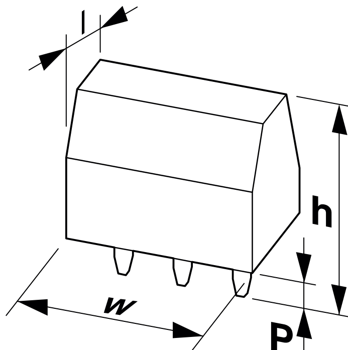
Rysunek wymiarowy
