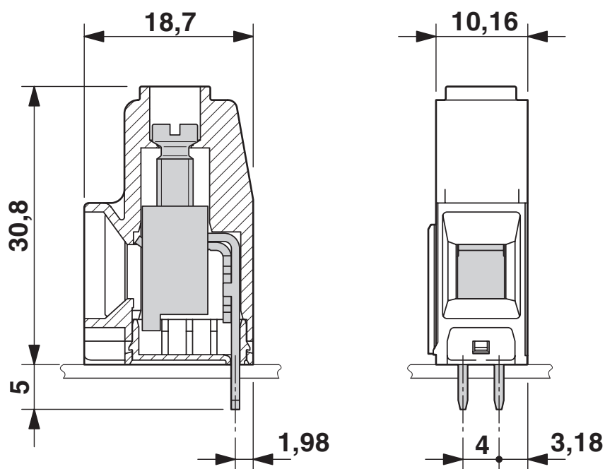
Rysunek wymiarowy
