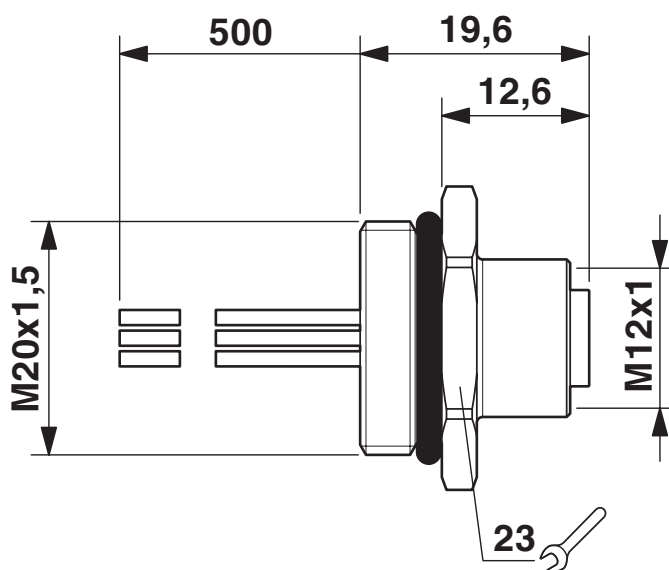
Rysunek wymiarowy
