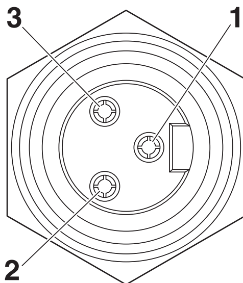
Rysunek schematyczny
