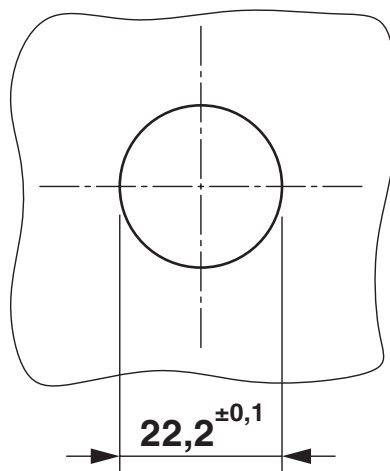
Rysunek wymiarowy
