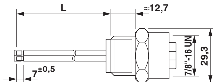
Rysunek wymiarowy
