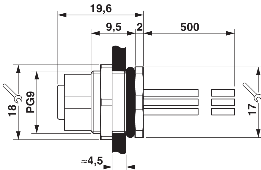
Rysunek wymiarowy
