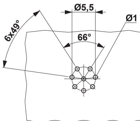
Otworowanie/geometria płytek lutowniczych
