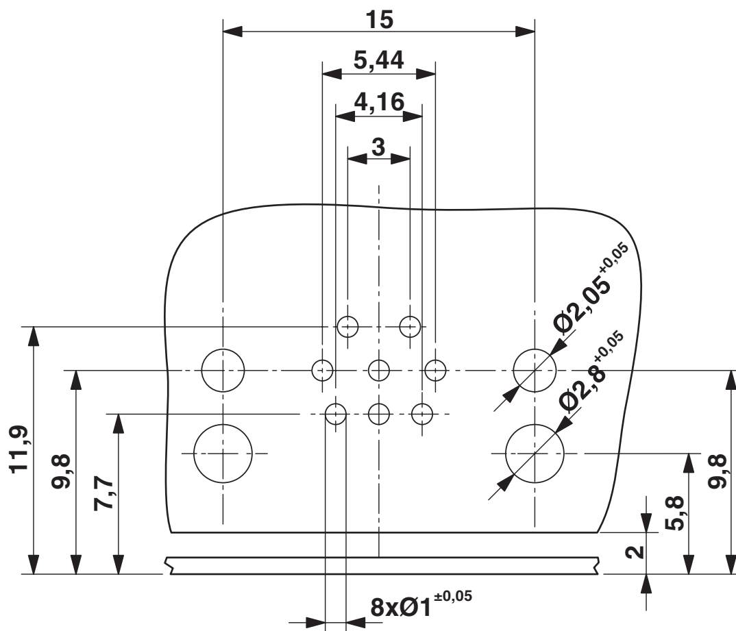
Otworowanie/geometria płytek lutowniczych
