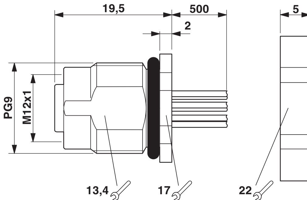
Rysunek wymiarowy
