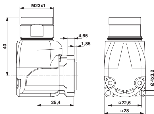
Rysunek wymiarowy
