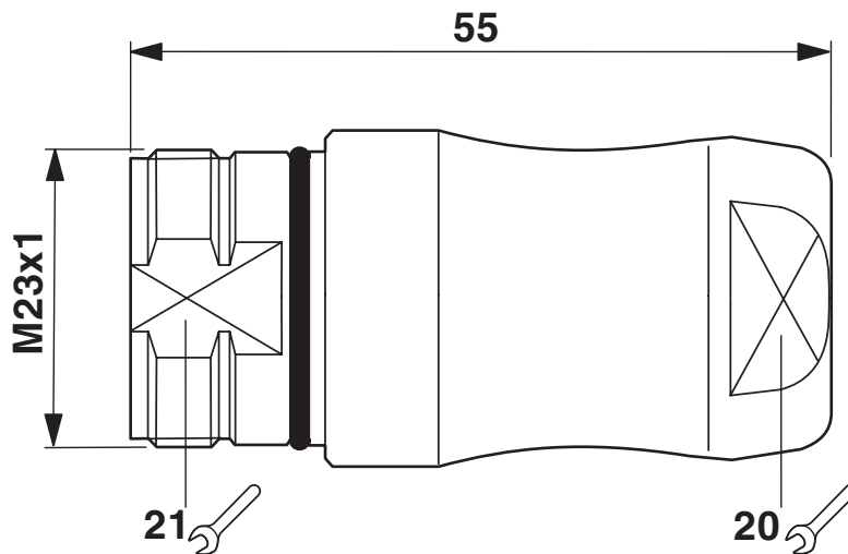
Rysunek wymiarowy
