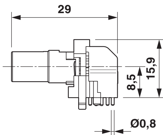
Rysunek wymiarowy
