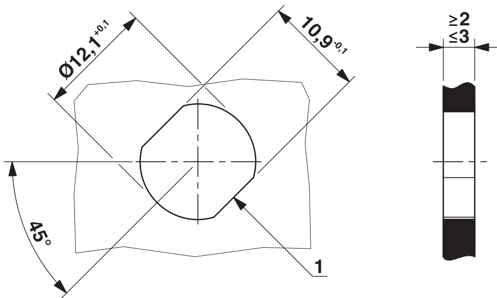
Fragment obudowy do gwintu mocującego M12, ściana montażowa z otworem przelotowym (alternatywnie z płaszczyznami zabezpieczającymi przed przekręceniem)
